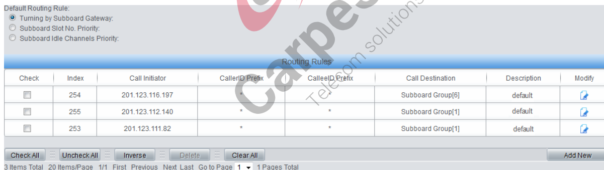
Рис. 3-13 Настройка параметров маршрутизации IP→TEL/PSTN
