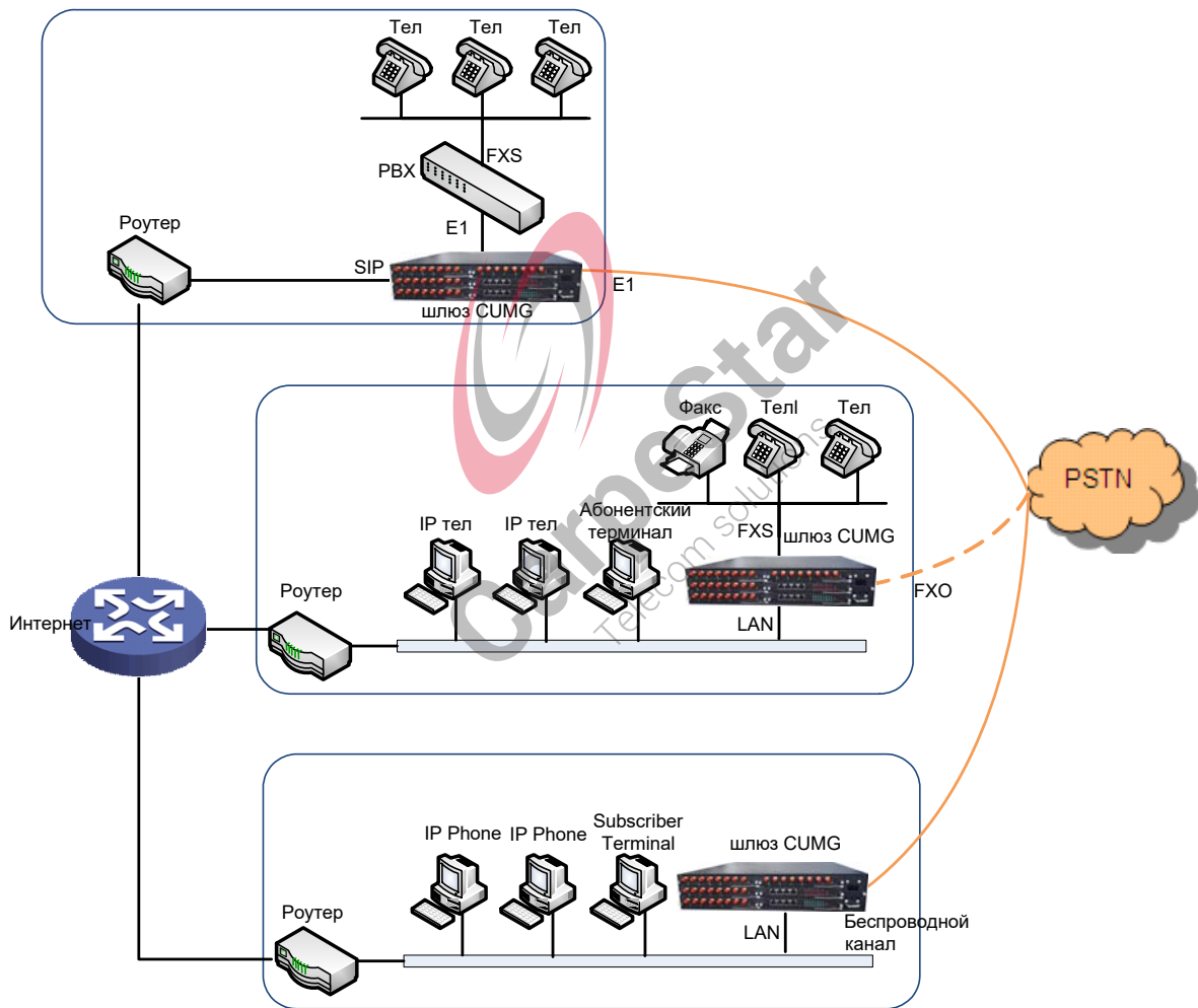
Рис 1-1 Типичное применение
