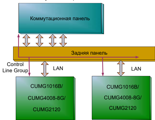
Рис 1-8 Архитектура шлюза CUMG Gateway
